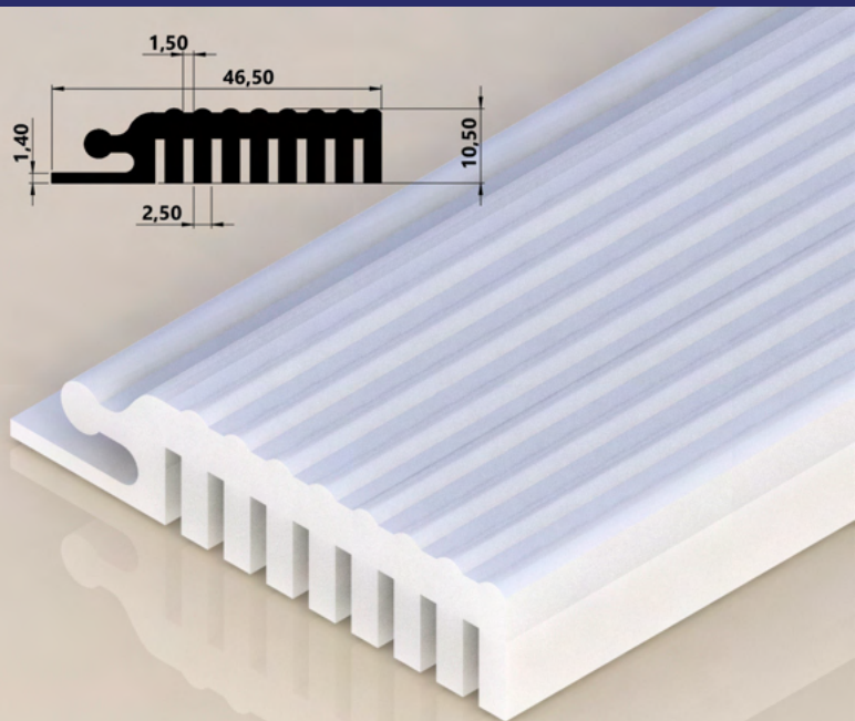
PERFIL GUIA 46,50X10,50MM
