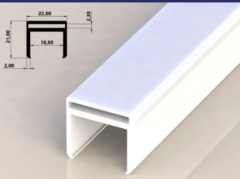
PERFIL TIPO U 22,80X21,00X2,00MM
