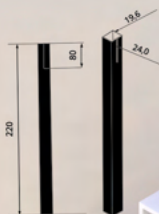
TUBO QUADRADO
