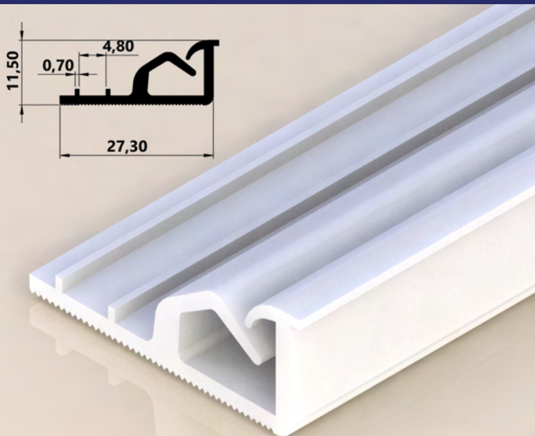
PERFIL RIGIDO 27,30X11,50MM
