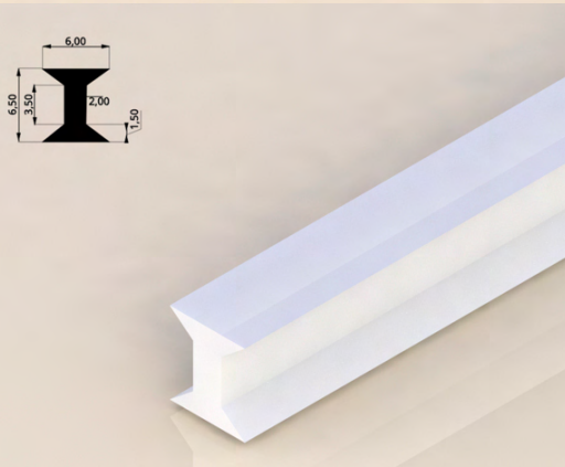
PERFIL DIVISORIA #1
