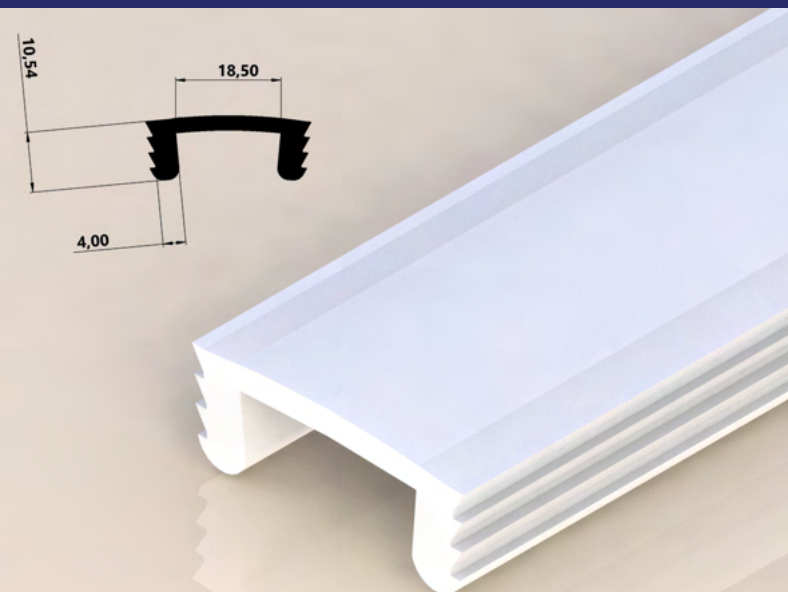
PERFIL JUNTA DE DILATAÇÃO 18,50X10,54X4,00MM
