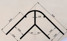
PERFIL QUADRADO COM ALETA 12 X 12MM
