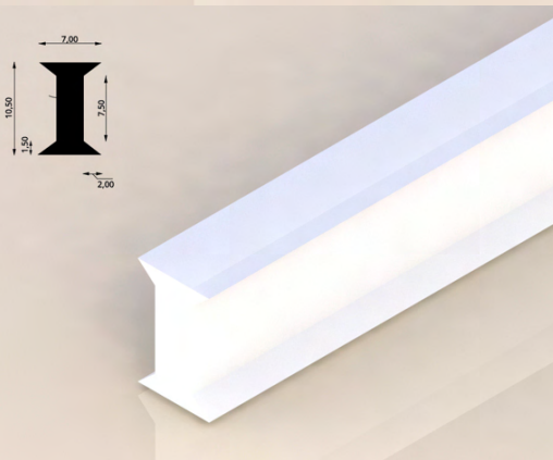
PERFIL DIVISORIA #3
