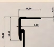
PERFIL TIPO BASE 115,45MM
