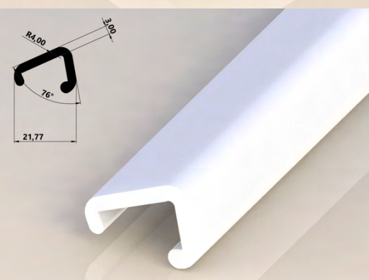
PERFIL TIPO ACABAMENTO 21,77 X 3,00MM
