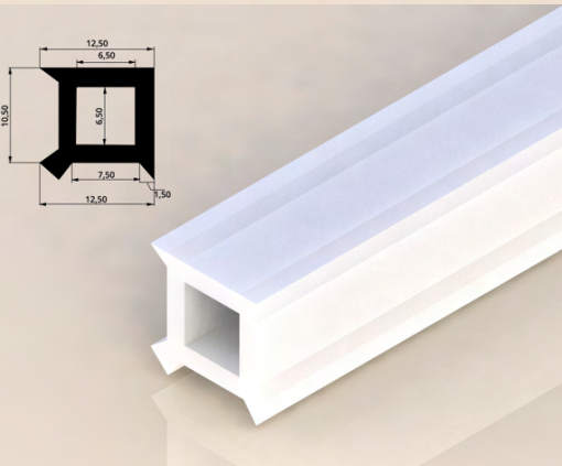
PERFIL DIVISORIA #2
